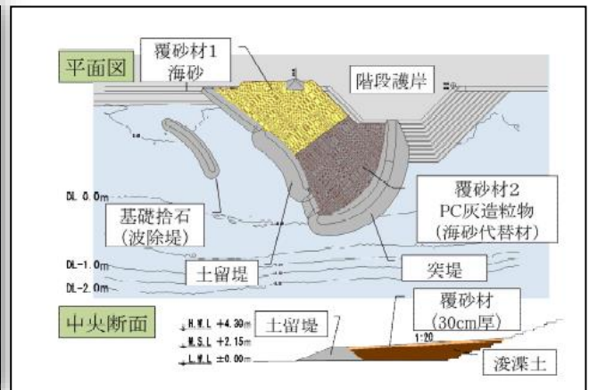
人工干潟「八代港なぎさ線」の概要 田中ら「人工干潟における生態系のモニタリング手法 に関する検討」(2014年)より
